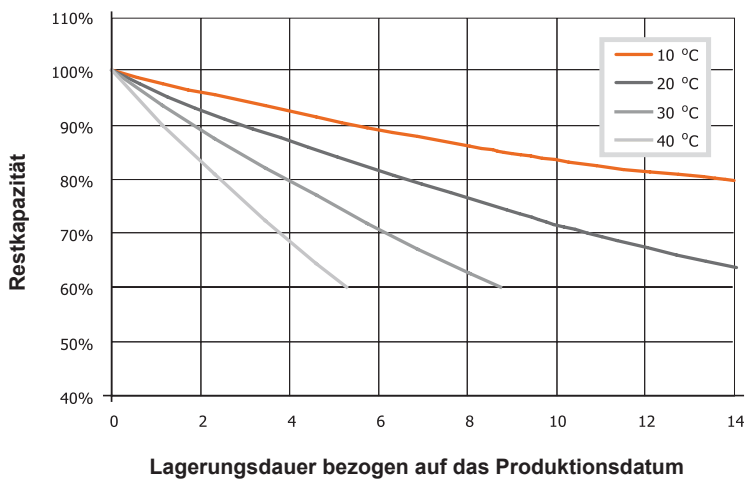
Selbstentladecharakteristik
